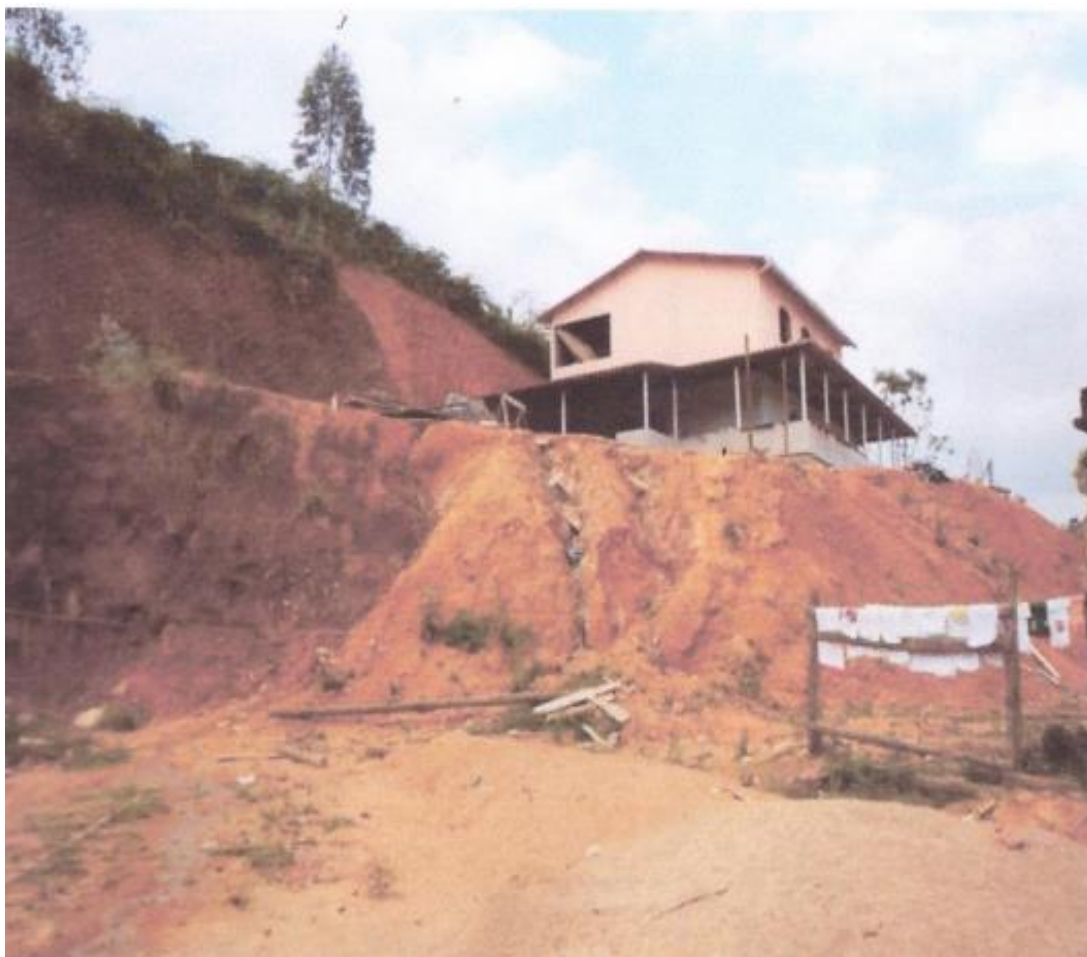
Foto 4: Imóvel em construção em corte e aterro.
